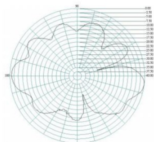
E-PLANE
